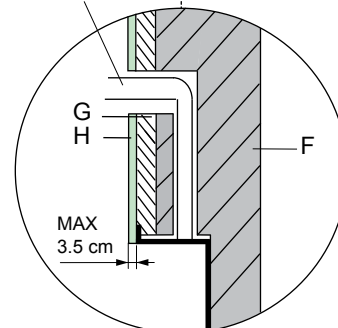
SOLUZIONE 2 Con cassa fissata sotto il rivestimento
