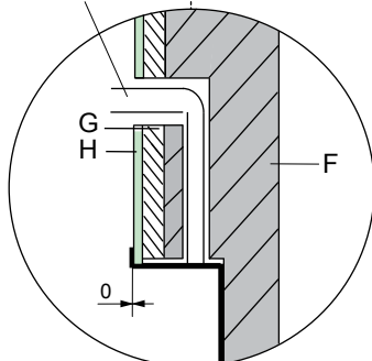
SOLUZIONE 1 Con cassa fissata sopra il rivestimento
